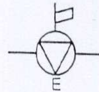
Robinet à eau pressostatique
