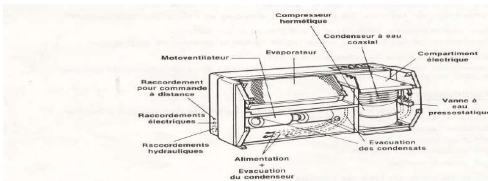
Figure 3 : climatiseur monobloc air/air
