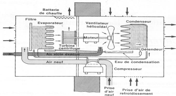
Figure 3 : climatiseur monobloc air/air
