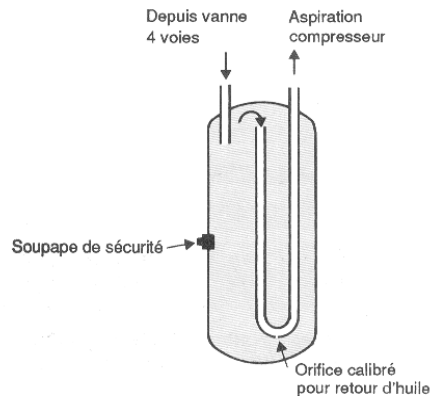
Figure 1 : bouteille anti coup de liquide
