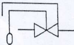
Detendeur thermostatique à égalisation externe de pression
