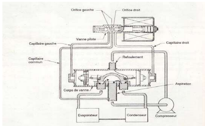
Figure 7 : vanne 4 vois bloquée (document RANCO)
