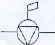
Robinet régulateur de pression à commande par le fluide lui-même
