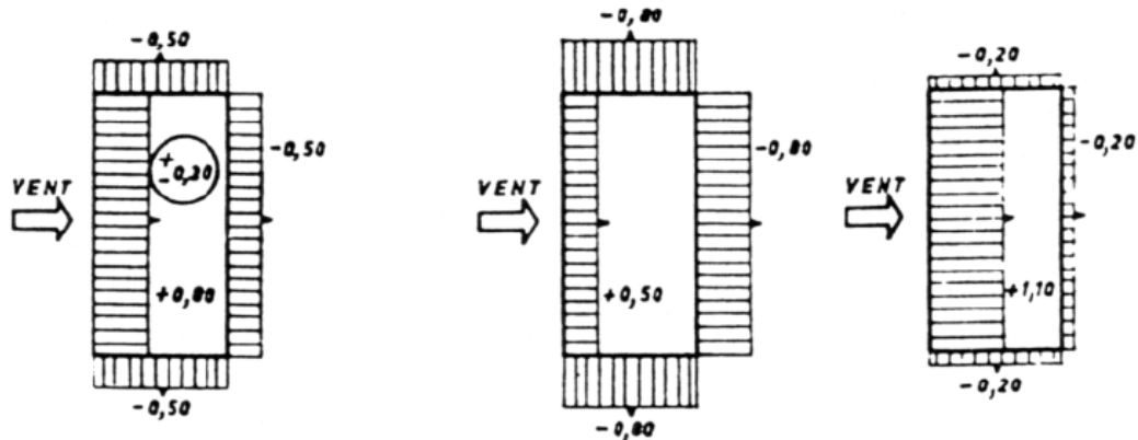
Dépression Intérieure de - 0,30
