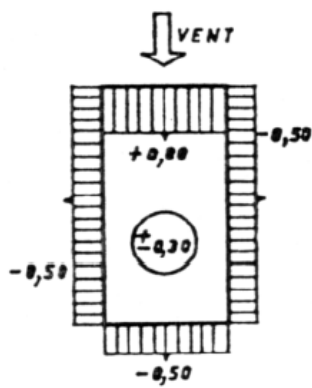
Actions extérieures et actions intérieures
