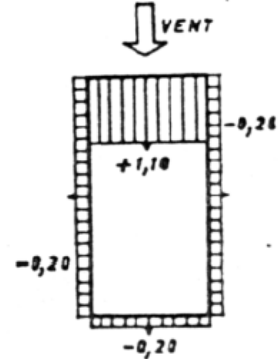
Dépression Intérieure de - 0,30
