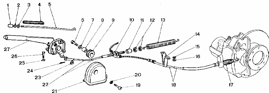
Fig.1 Vue éclatée du frein à main de secours et de stationnement.
