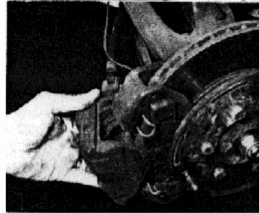
Fig 5: Dépose de l'étrier. (photo R.T.A)
