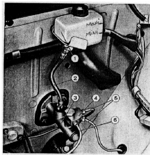
Fig 1. Réservoir et maître-cylindre de freins.
