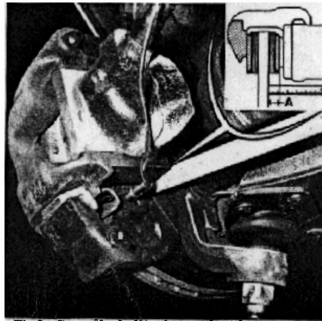
Fig 1: Contrôle de l'épaisseur des plaquettes avant sur véhicule. (Photo RTA).
