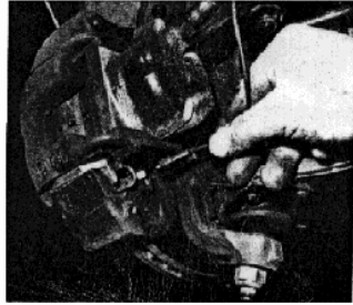
Débranchement du fil de témoin d'usure des plaquettes de freins avant. (photo RTA).
