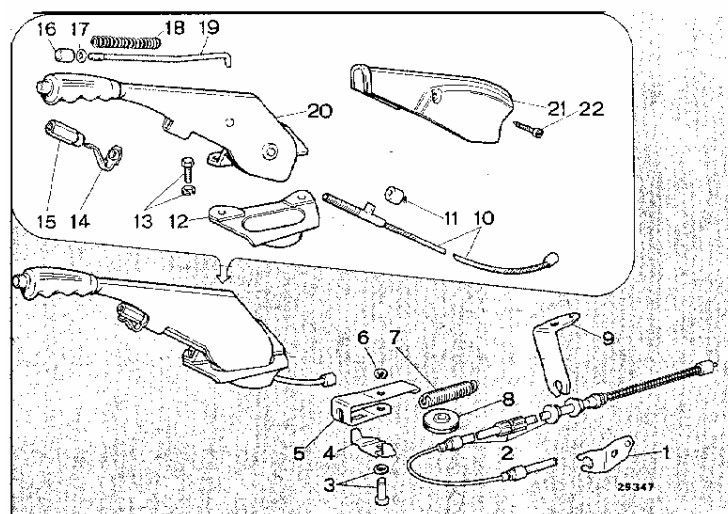
Fig.1 Composantes du frein à main
