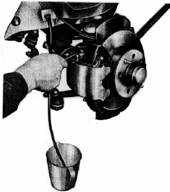
Fig.1 Purge d'air du circuit hydraulique de freinage de la roue AV droite.
