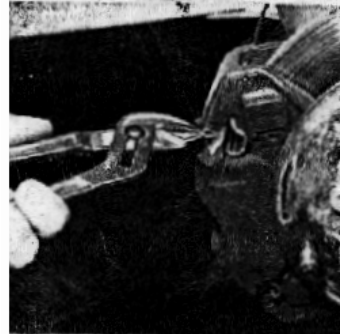
Débranchement du fil de témoin d'usure des plaquettes de freins avant. (photo RTA).
