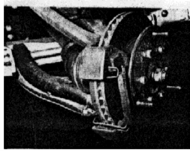
Fig 6 : Dépose des plaquettes, (photo R.T.A)
