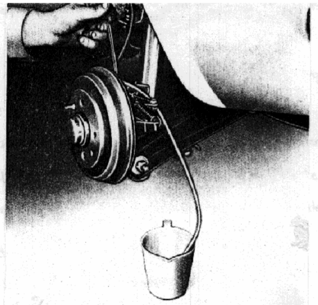
fig 2. Purge des canalisations du système hydraulique des freins à tambour.
