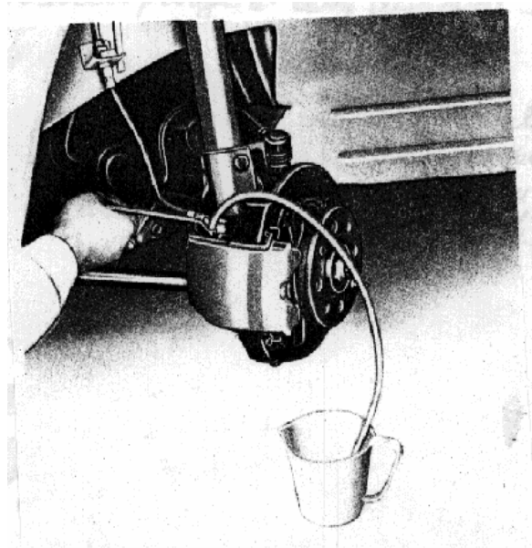
fig.1 Purge des canalisations du système hydraulique des freins à disque.
