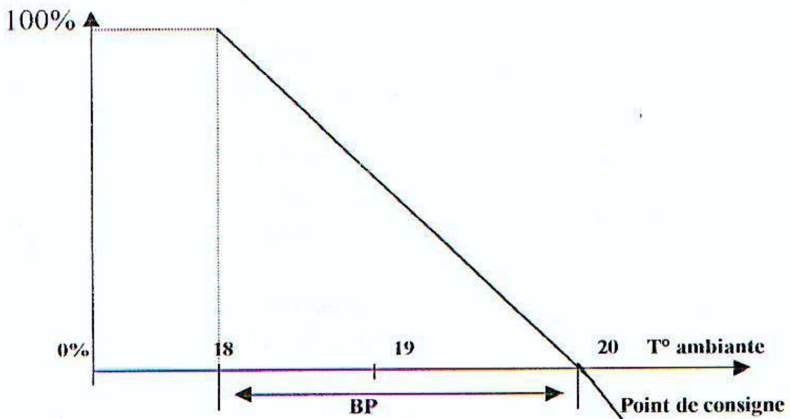
Fig.8 pente caractérisant la loi régulation Sur le schéma précédent on voit que : - le point de consigne est 20°e.
