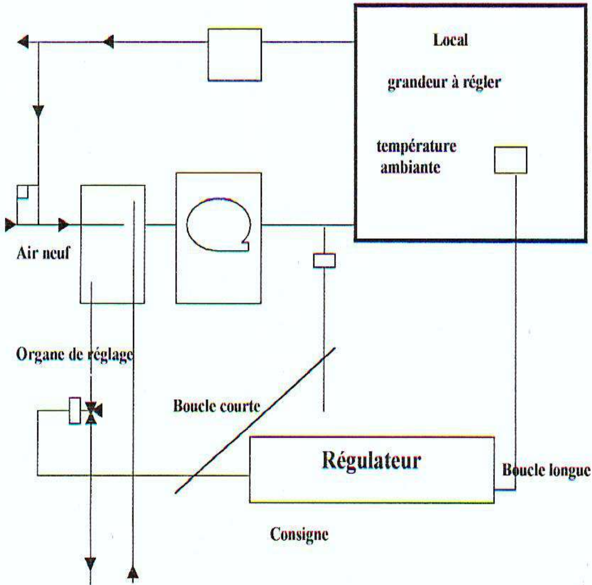
Fig.2 introduction d'une boucle courte
