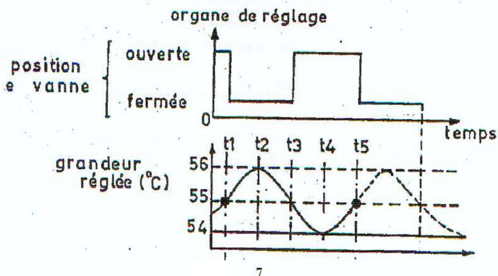
Fig.5 Régulation toute ou rien
