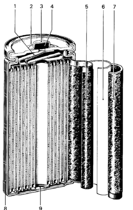
Accumulateur alcalin
