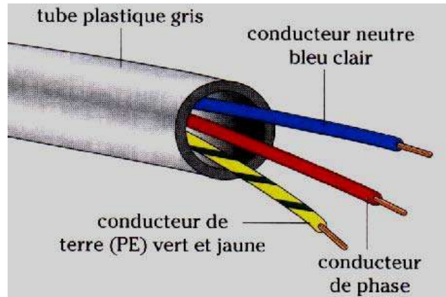
Figure 4.1 - Canalisation électrique
