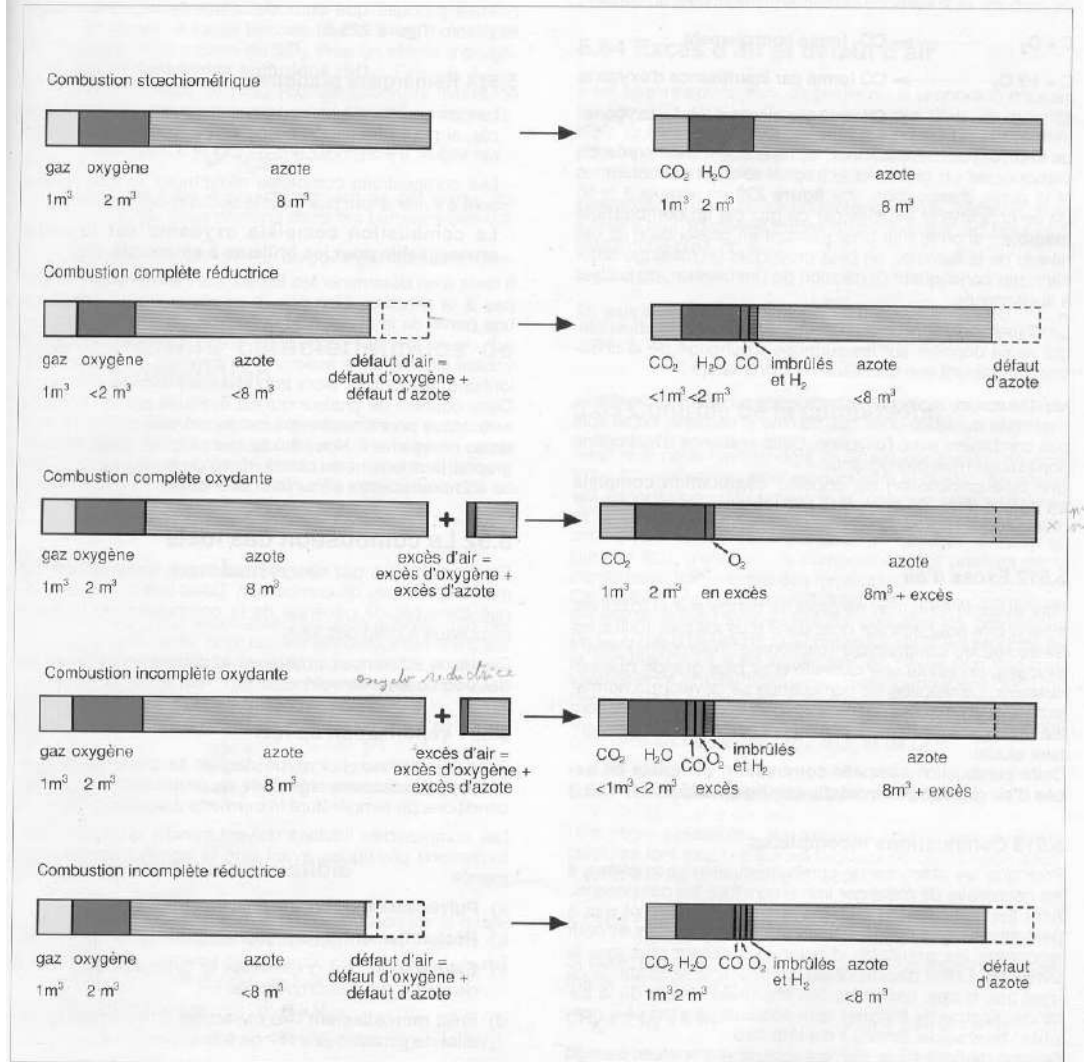
Figure 225. Représentation simplifiée de la combustion d'un mètre cube de méthane
