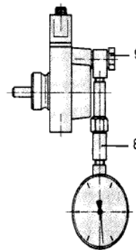
Raccordement manomètre
