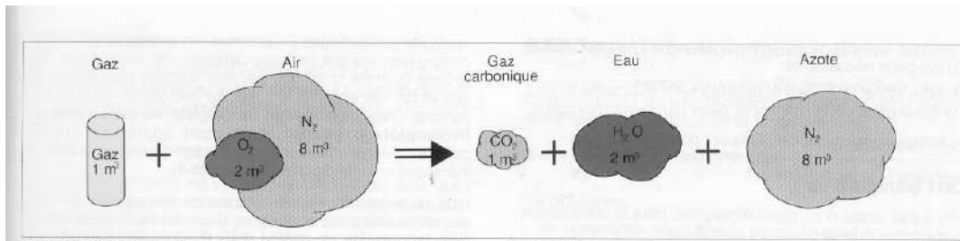
Figure 225. Représentation simplifiée de la combustion d'un mètre cube de méthane
