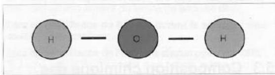
Représentation symbolique d'une molécule d'eau.
